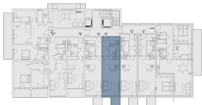
Půdorys podlaží
