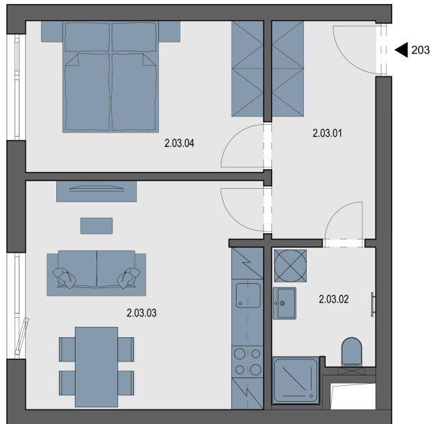
Půdorys podlaží
