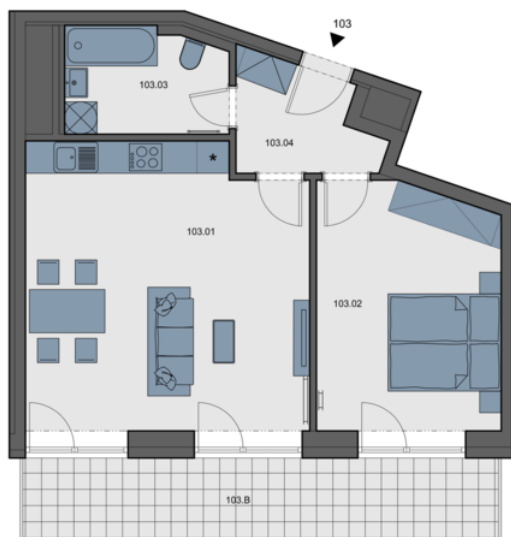
PŮDORYS PODLAŽÍ
