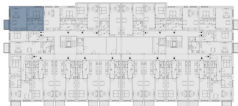
PŮDORYS PODLAŽÍ
