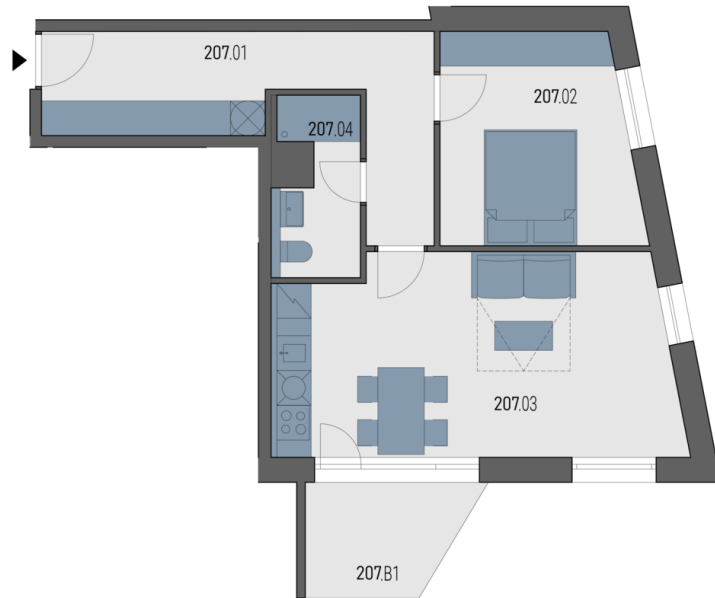
Půdorys podlaží
