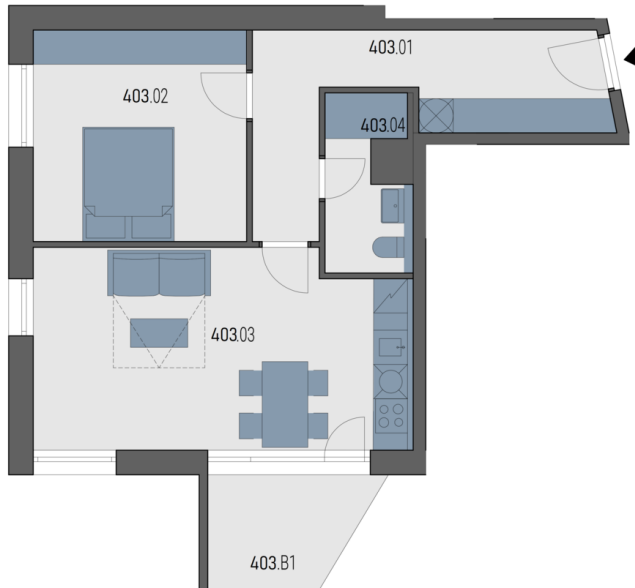
Půdorys podlaží
