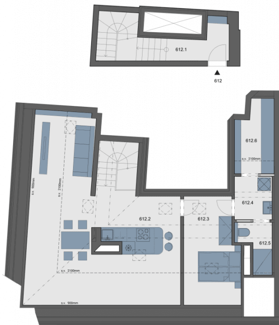
ПЛАН ЭТАЖА
