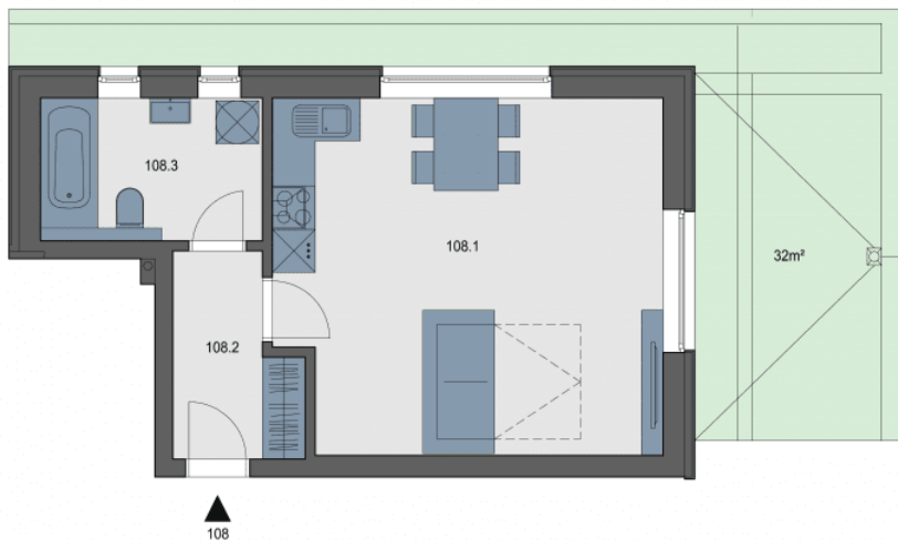
ПЛАН ЭТАЖА
