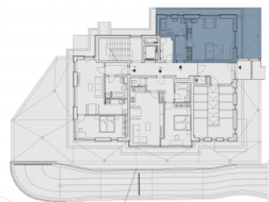
ПЛАН ЭТАЖА
