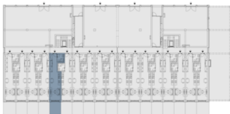
ПЛАН ЭТАЖА
